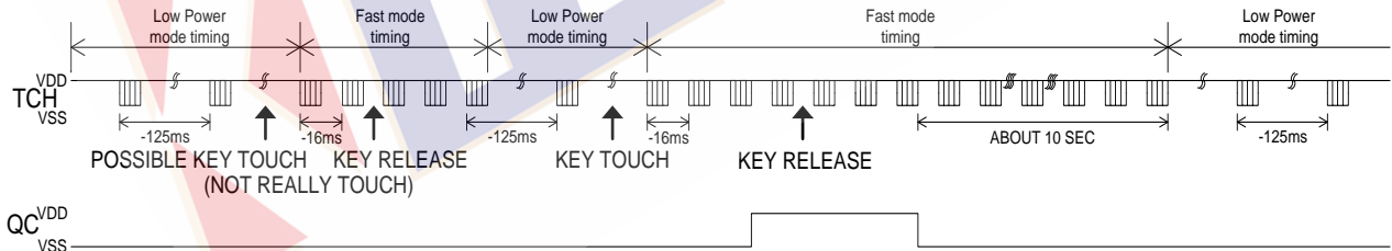
图 5 时序图
