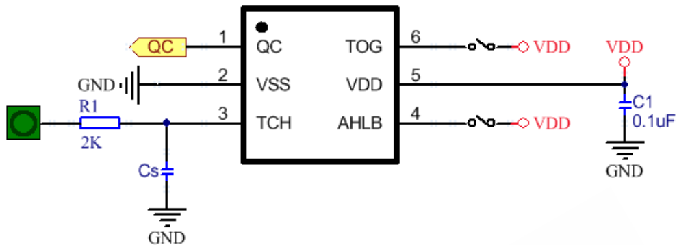
图 6 电路示意图
