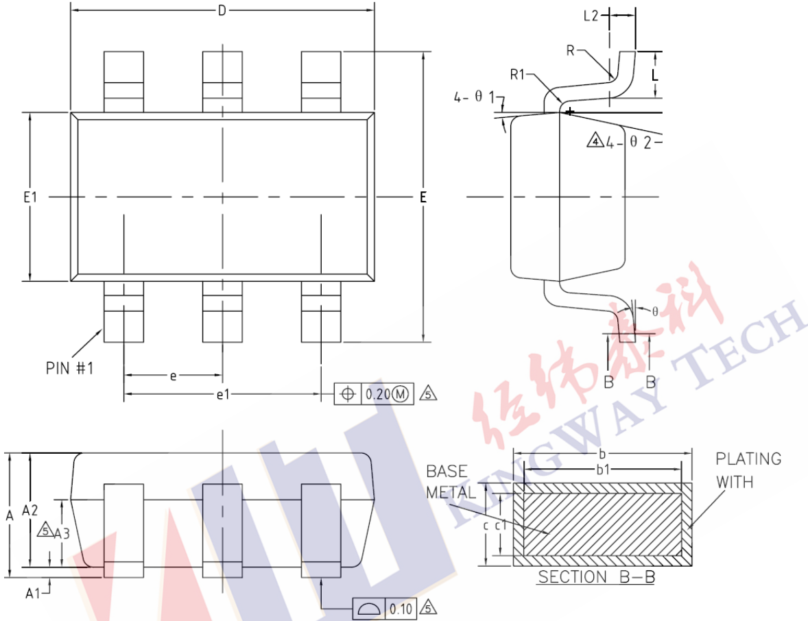
图 7 SOT23-6 封装图
